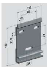
Placa Frontal
